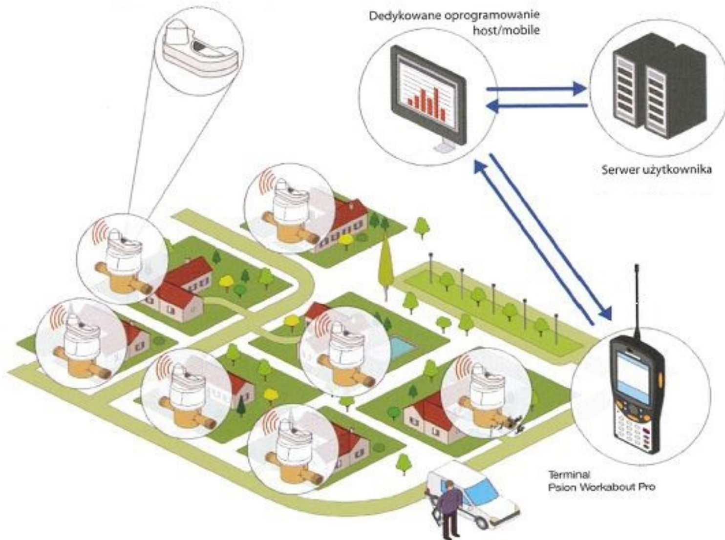
Radiowy dwukierunkowy system odczytu wodomierzy
